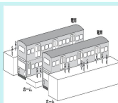
総2階建て車両と対応する駅構造 「満員電車がなくなる日」より
